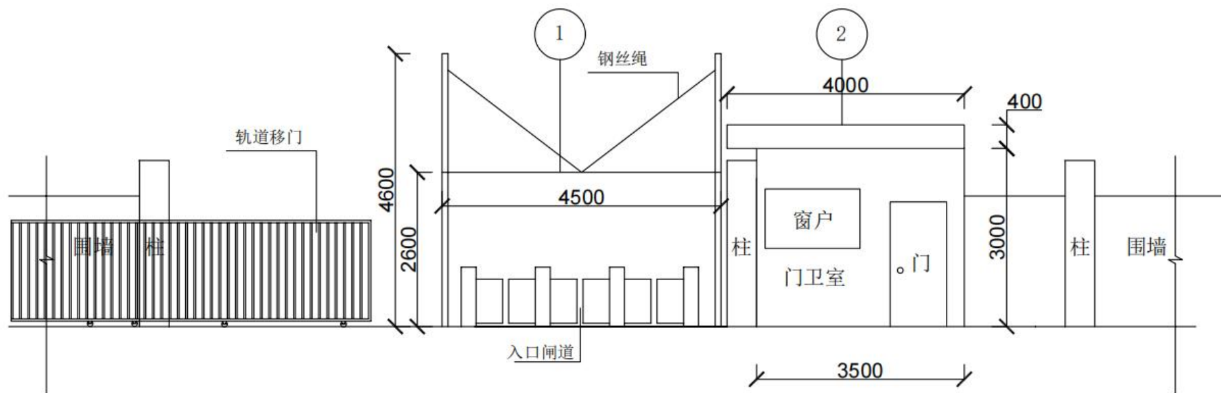
西门大门设计
