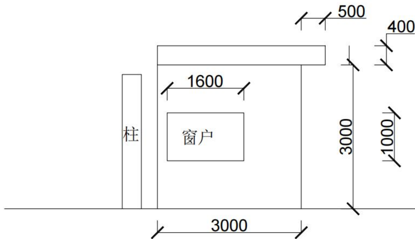
② 门卫室侧面图
