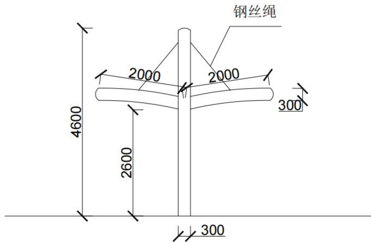
① 遮阳棚侧面图
